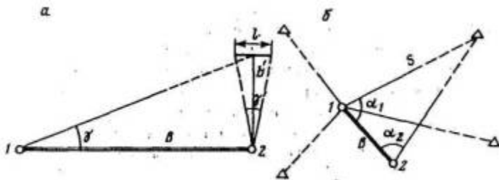
Рис. 37. Схемы определения длины базиса фотографирования: а) с помощью вспомогательного базиса; б) из неполного треугольника
