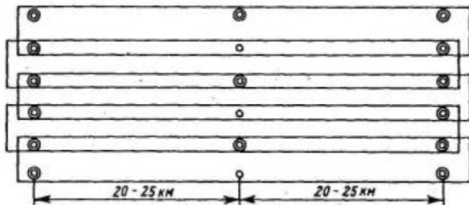
Рис. 7. Съёмка в масштабе 1:25 000 с сечением рельефа через 5,0 м
