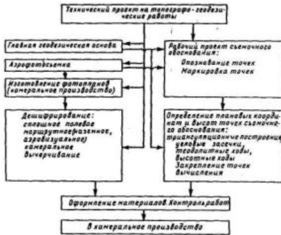
Рис. 1. Технологическая схема полевых работ при стереотопографической съемке
