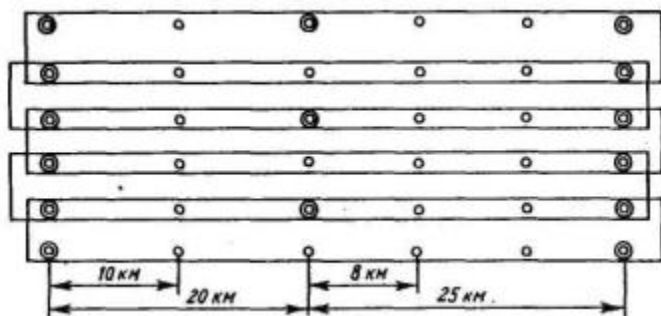
Рис. 6. Съёмка в масштабе 1:25 000 с сечением рельефа через 2,5 м
