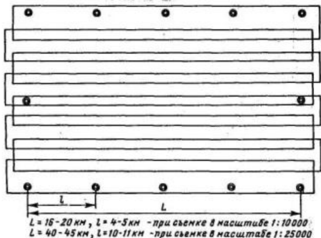
Рис. 9. Схема съемочного обоснования блока
